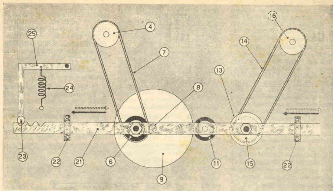
Fig. 2. - 4) Rullo di 24 mm. di diametro, sottostante il PORTABOBINA 1. — 6) Rullo di gomma fissato alla piastra n. 21, diametro mm. 24. — 7) Cinghia di trasmissione in gomma o a molla. — 8) Perno con boccia, diametro, 6 mm. — 9) Rullo di metallo fissato al perno n. 8. — 11) Rullo del motorino. — 13) Rullo di metallo fissato al perno n. 12. — 14) (Vedi part. 7). — 15) Rullo di metallo con scanalatura. — 16) (Vedi part. 15). — 21) Asta metallica, spessore 2 mm., larghezza 15 mm. — 22) Guide metalliche per il part. 21. — 23) Rotella appartenente al dispositivo d'arresto, spessore mm. 5. — 24) Molla del dispositivo d'arresto. — 25) Leva azionante la rotella d'arresto. Il dispositivo d'arresto va fissato sullo stesso piano dell'asta mobile.
